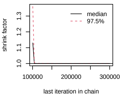
d.I.I_IGF_1Ri
