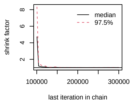
d.I.I_HGFi
