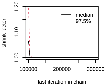
d.I.Placebo
