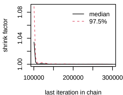
d.I.I_METi
