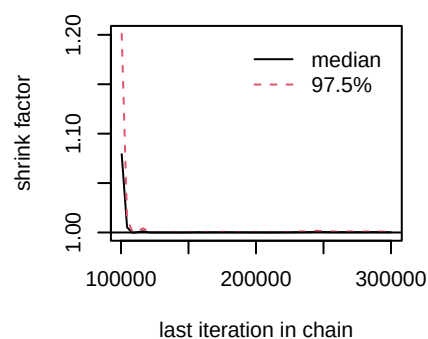
d.III.III_antiangio
