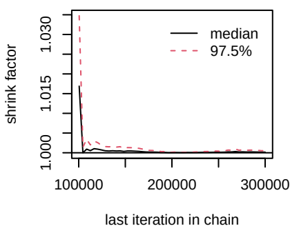
d.I.I_chemo
